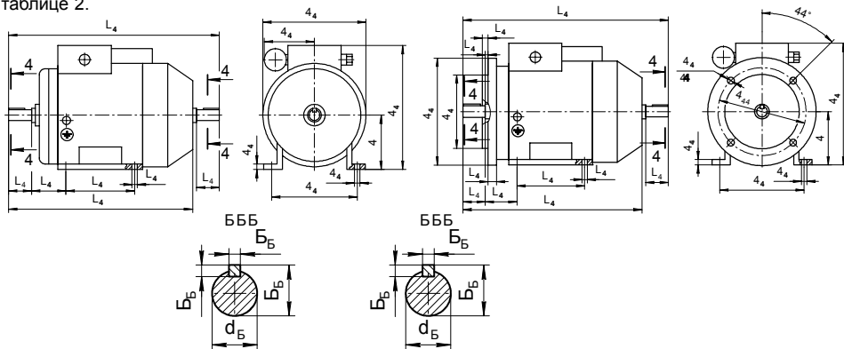
Рисунок 2 – Габаритные, установочные и присоединительные размеры
