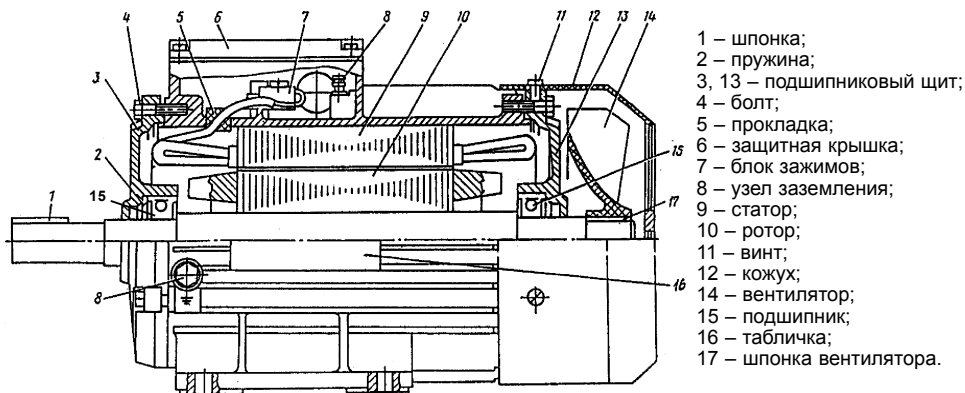
Рисунок 1 – Устройство двигателя
