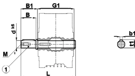
Односторонний выходной вал
