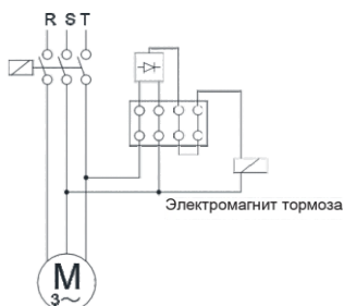
Тормоз с задержкой включения (220 В)
