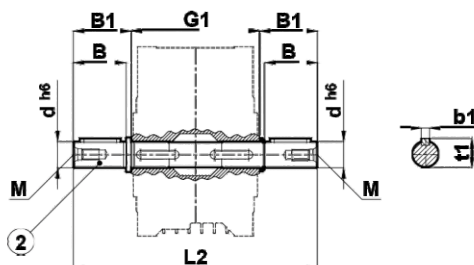
Двухсторонний выходной вал
