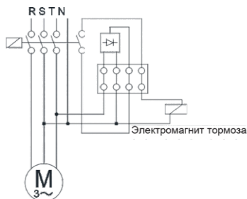
Тормоз без задержки включения (220 В)
