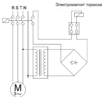
Тормоз без задержки включения (24 В)
