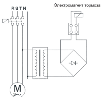
Тормоз с задержкой включения (24 В)
