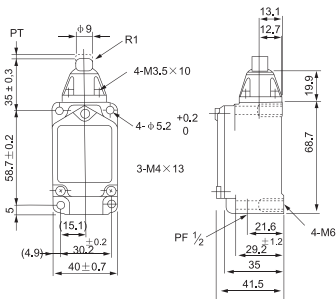
Рис. 4 - Габаритные размеры концевых выключателей WLCL EKF
