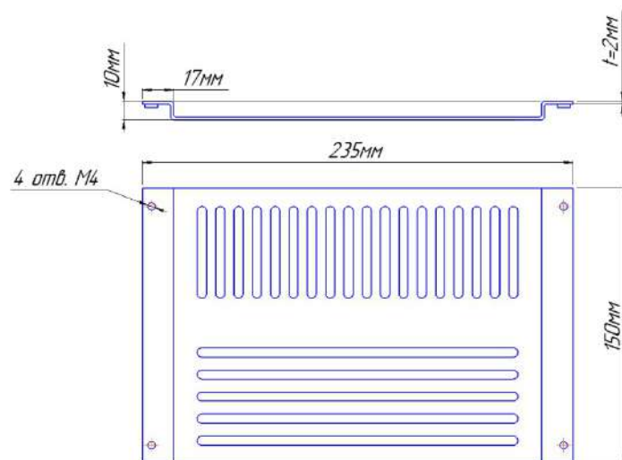
Чертеж 2. Габаритные размеры Н0-ZA2
