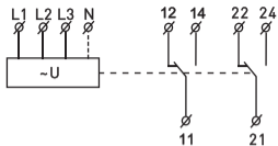
Рис. 4 – Схема подключения реле
