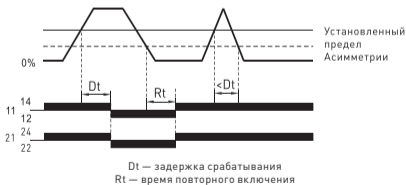
Рис. 3 – Принцип работы реле при асимметрии напряжения
