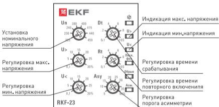
Рис. 5 – Основные элементы реле
