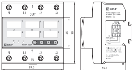
Рис. 15 - Габаритные и установочные размеры
