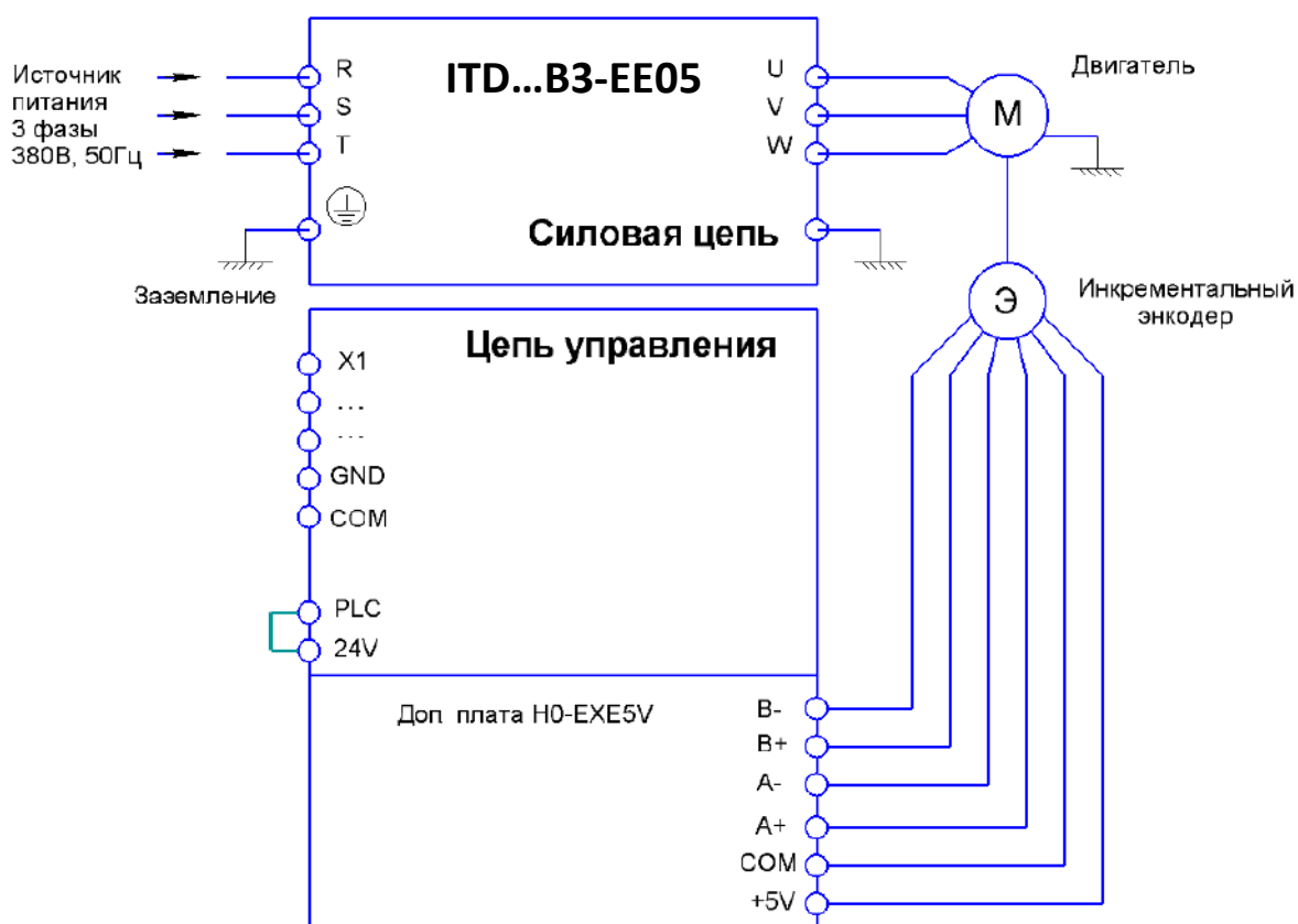
Электрическая схема подключения платы
