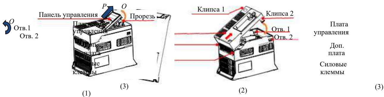
Рис.2-8 (а) ITD...B3 (1.5~11кВт)
