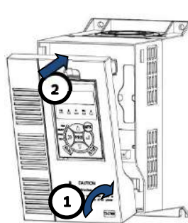
Рис.2-7 Снятие пластикового корпуса
