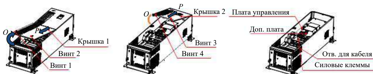
Рис.2-10 ITD...B3 (160~315 кВт)
