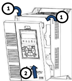
Рис.2-6 Установка пластикового корпуса
