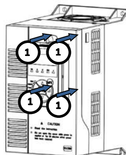
Рис.2-5 Установка клавиатуры
