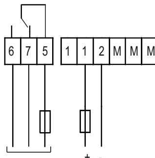
Выходной сигнал Источник питания
