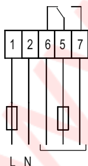
Источник питания Выходной сигнал
