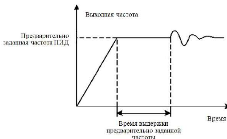
Рис. 6-24 Предварительно заданная частота и время выдержки предварительно заданной частоты ПИД
