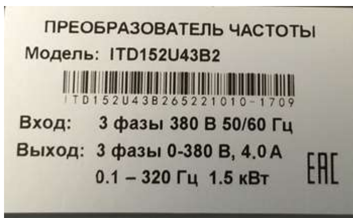
Рис.1-2 Заводская табличка
