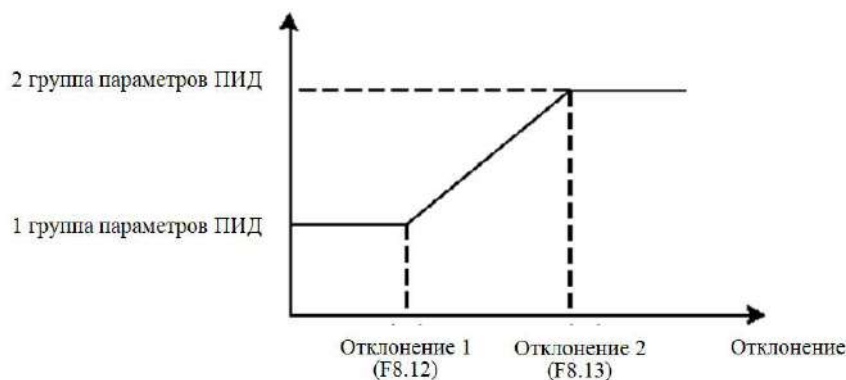
Рис. 6-23 Переключение параметров ПИД
