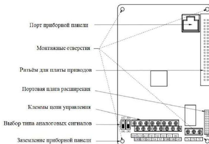
Рис. 3-20 Плата управления
