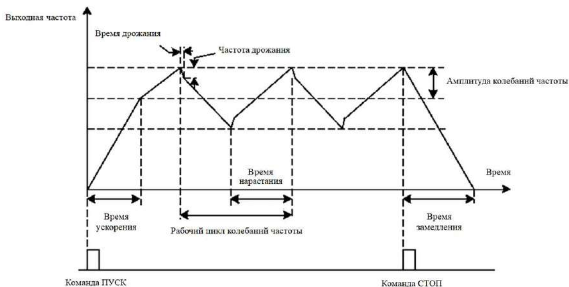
Рис. 6-26 Схема изображения колебаний частоты
