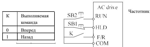
Рис.6-16 Трехпроводной режим управления 2
