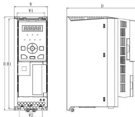
Рис. 1. IMD_E 0,75 – 5,5 кВт
