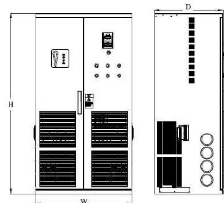
Рис. 6. IMD_E 500 – 710 кВт
