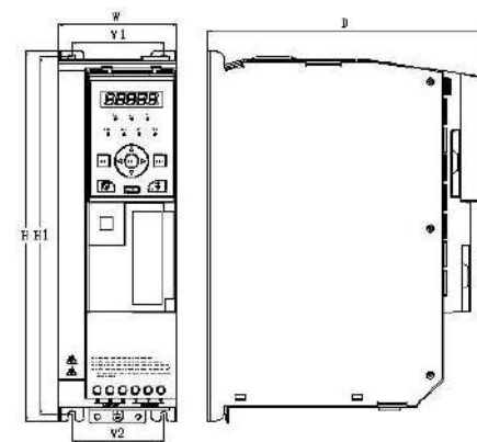
Рис. 2. IMD_E 7,5 – 15 кВт
