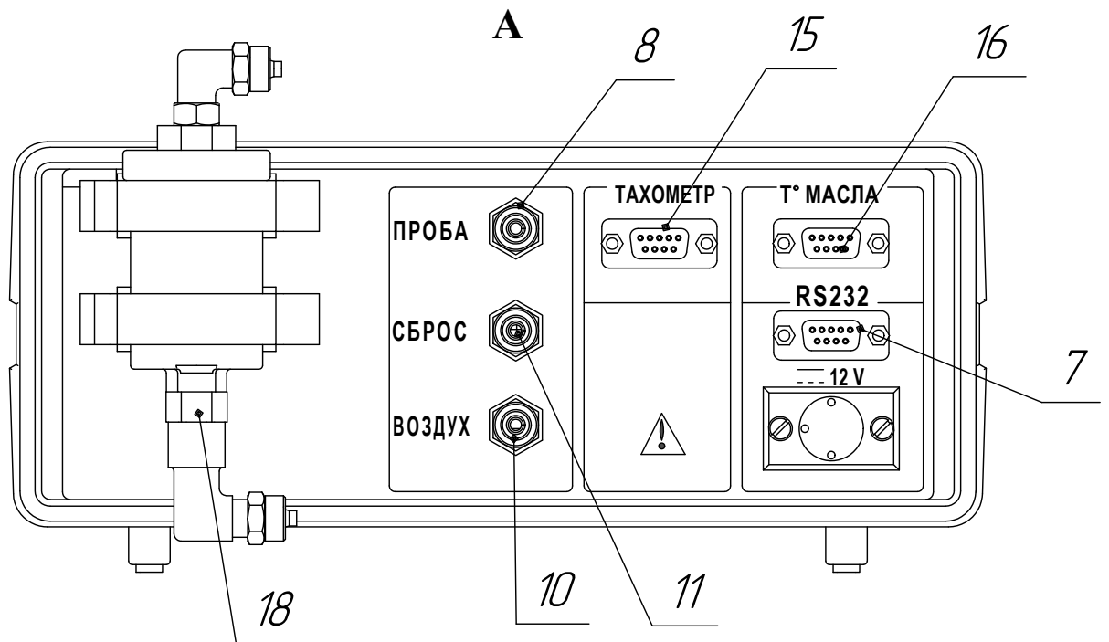
Рисунок 1.1б - Газоанализатор ГИАМ-29М-2. Внешний вид
