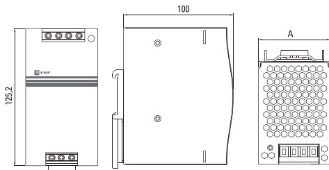
Рис. 4 Габаритные размеры блока питания DR-75W-24, DR-120W-24, DRP-240W-24.
