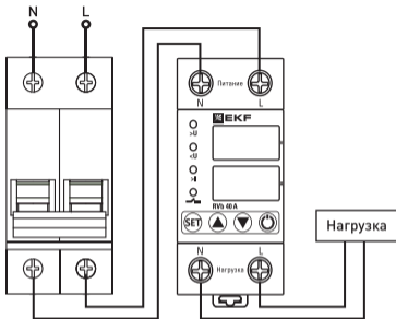
Рис. 5 – Схема подключения
