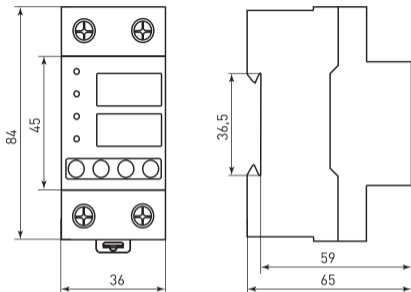
Рис. 6 – Габаритные размеры
