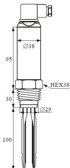
Рис.1 Размеры и тип электрического подключения
