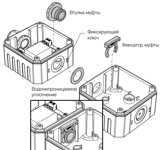
Кабельный сальник
