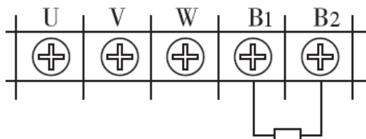
Тормозной резистор
