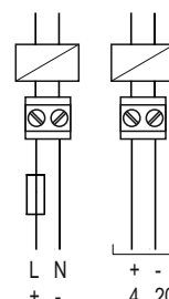
Выход 4...20 мА
