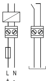
Выход реле
